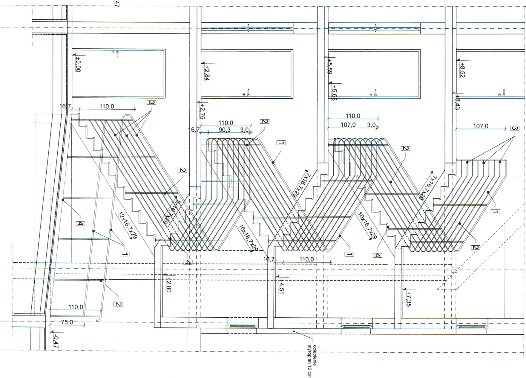
BALUSTRADA B1 KLATKI SCHODOWEJ
